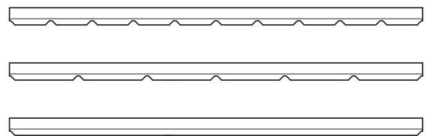
Tværsnit af Troldtekt v-line 2way 6, v-line 2way 10 og v-line 2way blank. Plademål: 25 x 600 x 1200 mm.
