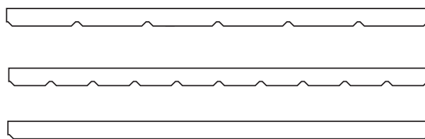
Tværsnit af Troldtekt v-line 1way 6, v-line 1way 10 og v-line 1way blank. Plademål: 25 x 600 x 1200 mm.
