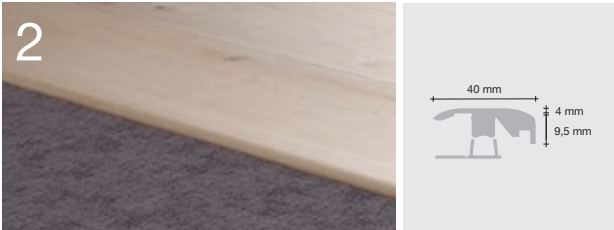
Overgangsprofil Fra laminat til tæppe.
