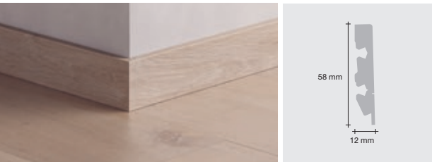
Farvematchet fodliste PGSK(-), 2400 × 12 × 58 mm*
