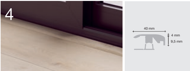
Afslutningsprofil Afslutning op mod dørtrin, skydedøre osv.
