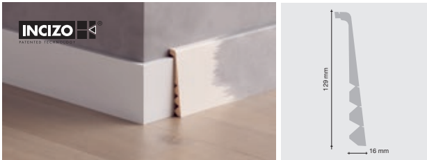
Fodliste, dækning PGISKRCOVER, 2400 × 16 × 129 mm
