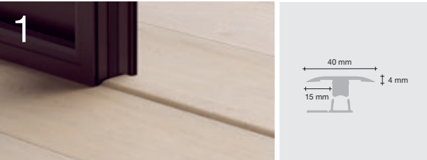
Ekspansionsprofil Fra laminat til laminat.
