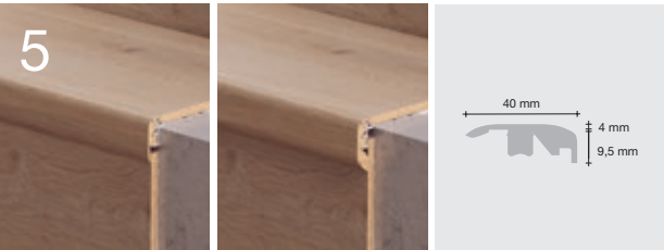
Trappeforkantsprofil, niveau For en flugtende afslutning på trappetrin.
