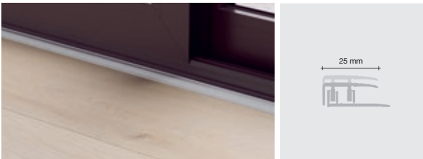
Afslutningsliste PGENPSILVME270, 2700 × 25 mm
