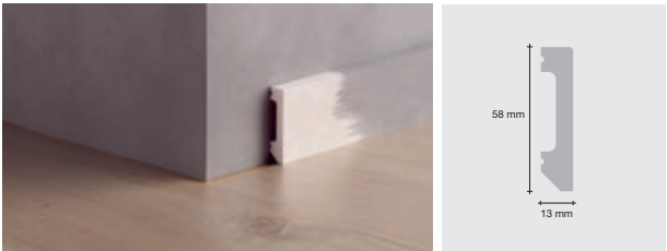
Vandtæt og malbar fodliste PGHSK58PAINT, 2400 × 13 × 58 mm
